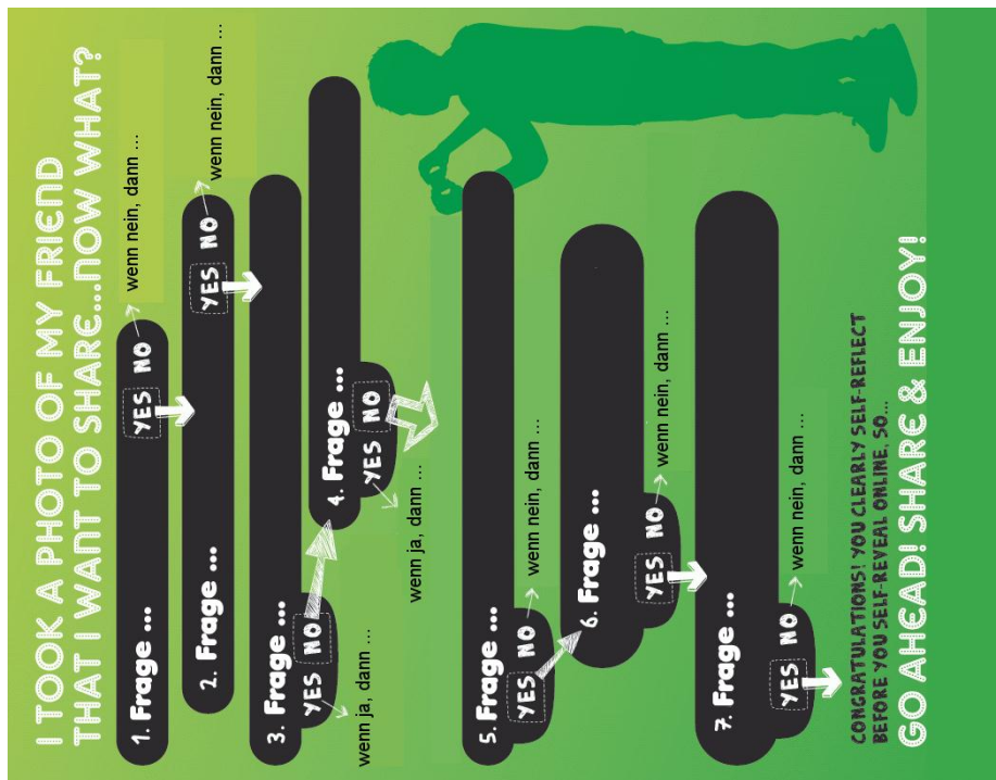
Beispiel Entscheidungsbaum
